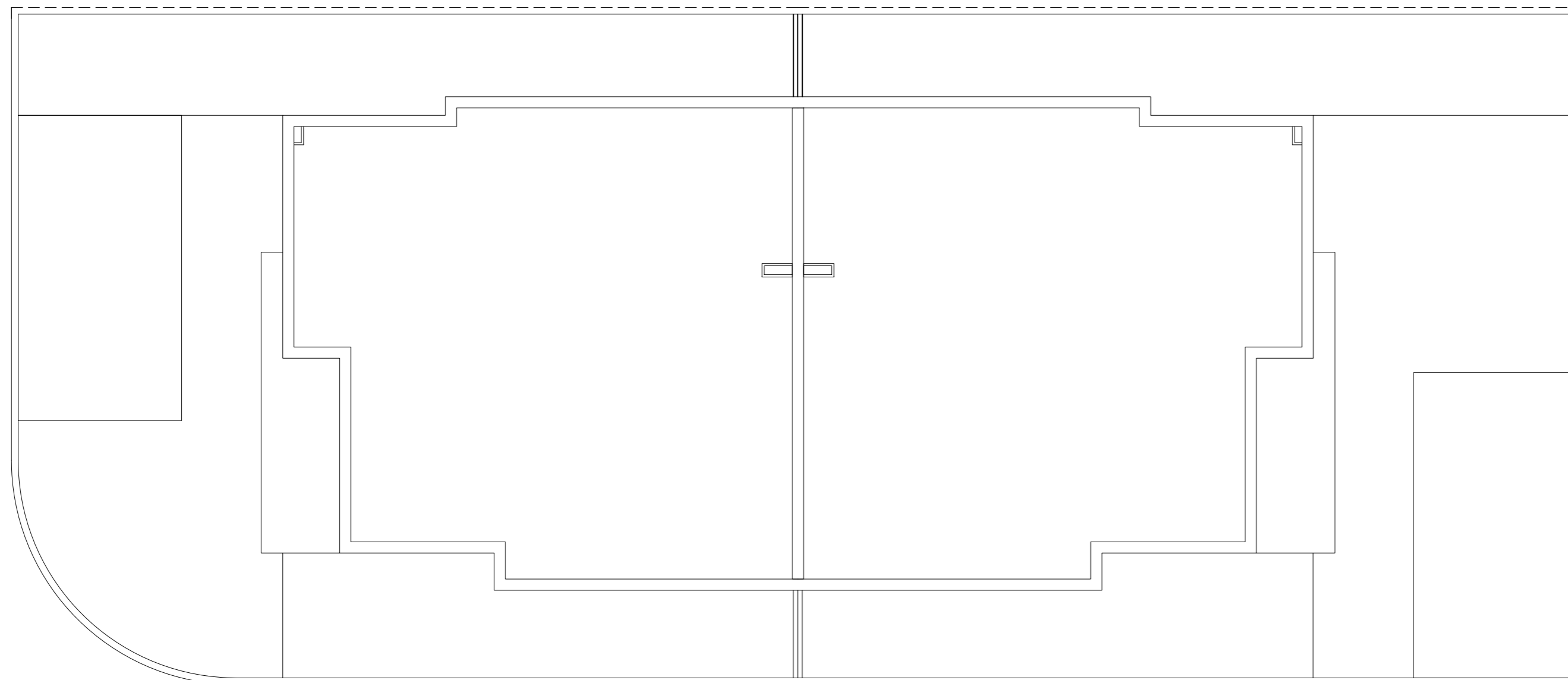
PLANTA CUBIERTAS VIVIENDAS 9 Y 10
