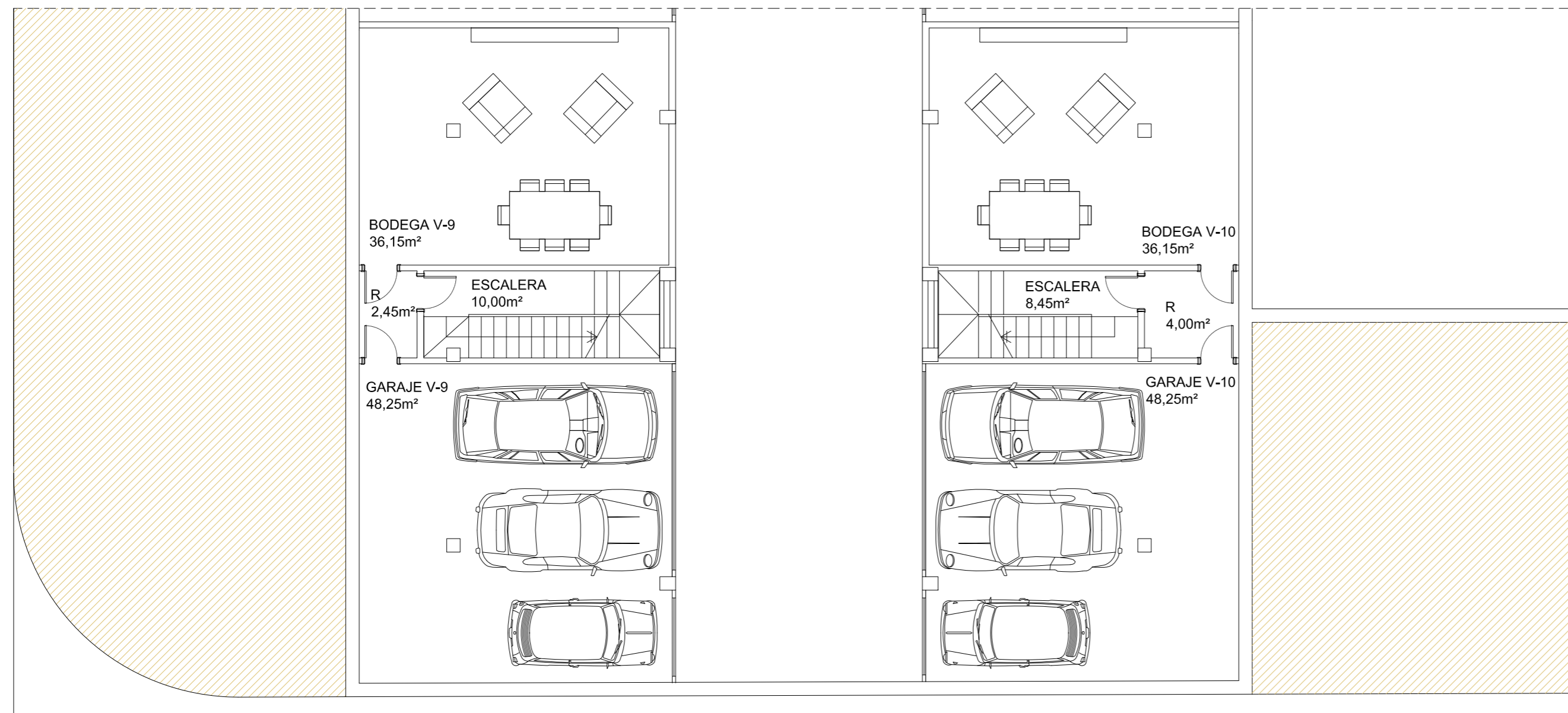
PLANTA SOTANO VIVIENDA 9 Y 10
