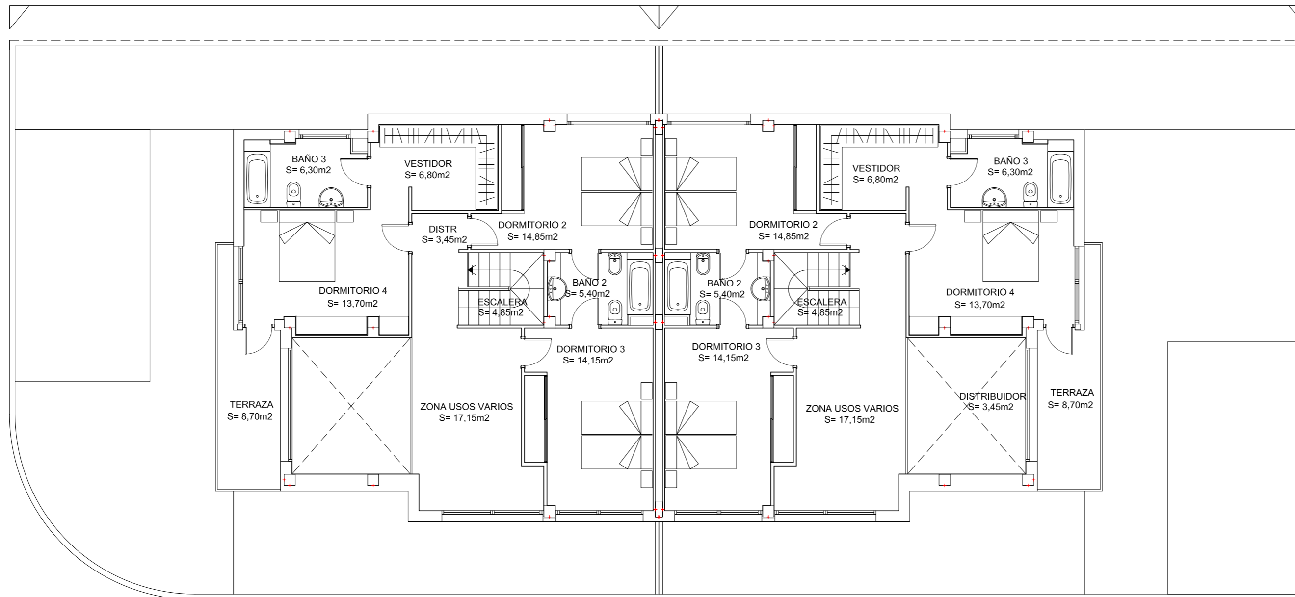
PLANTA PRIMERA VIVIENDAS 9 Y 10
