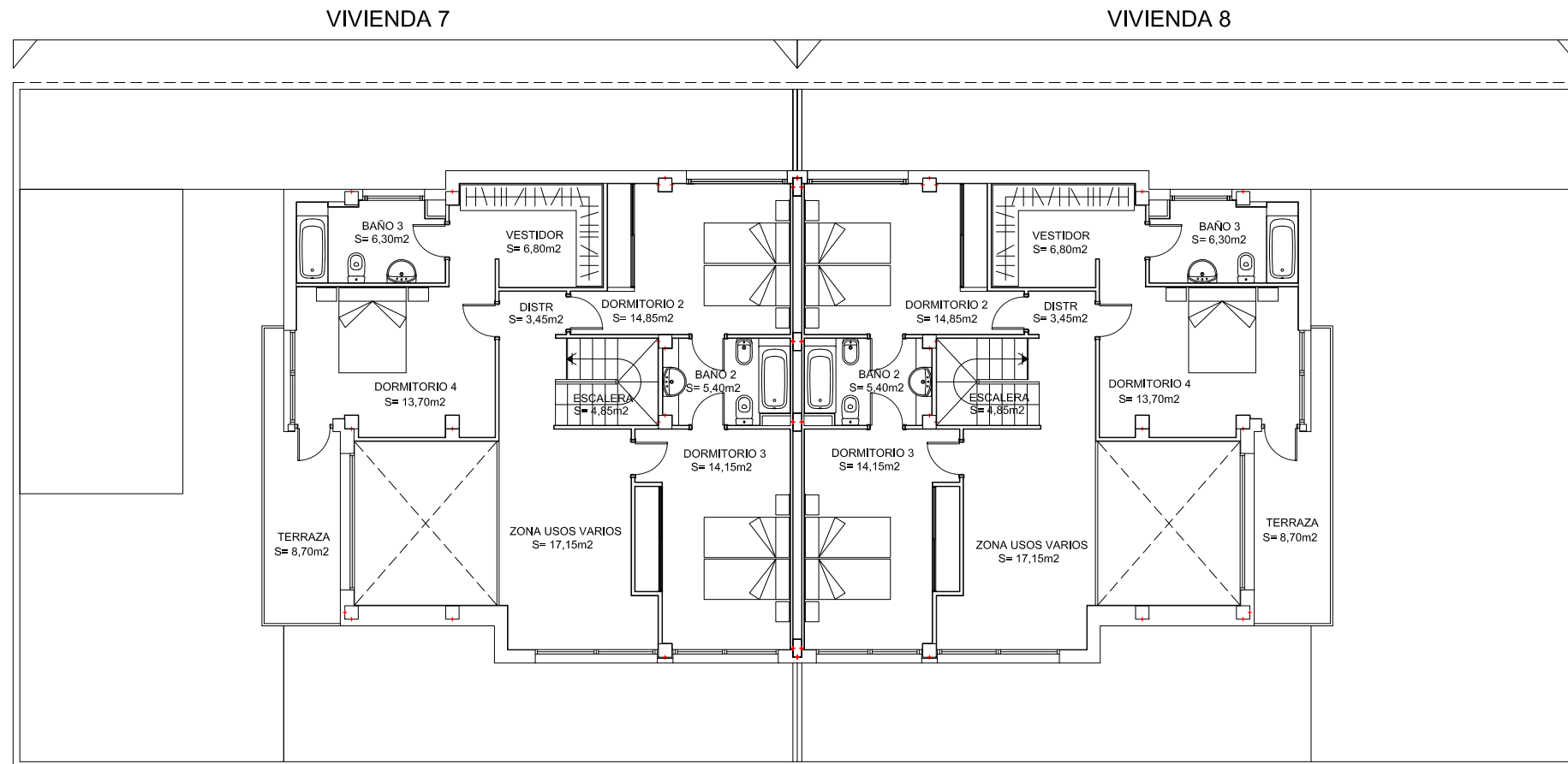
PLANTA PRIMERA VIVIENDAS 7 Y 8
