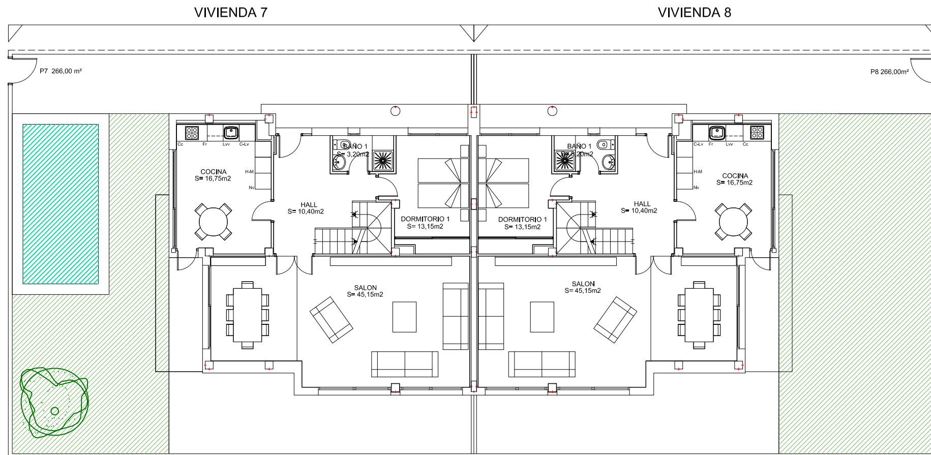
PLANTA BAJA VIVIENDAS 7 Y 8
