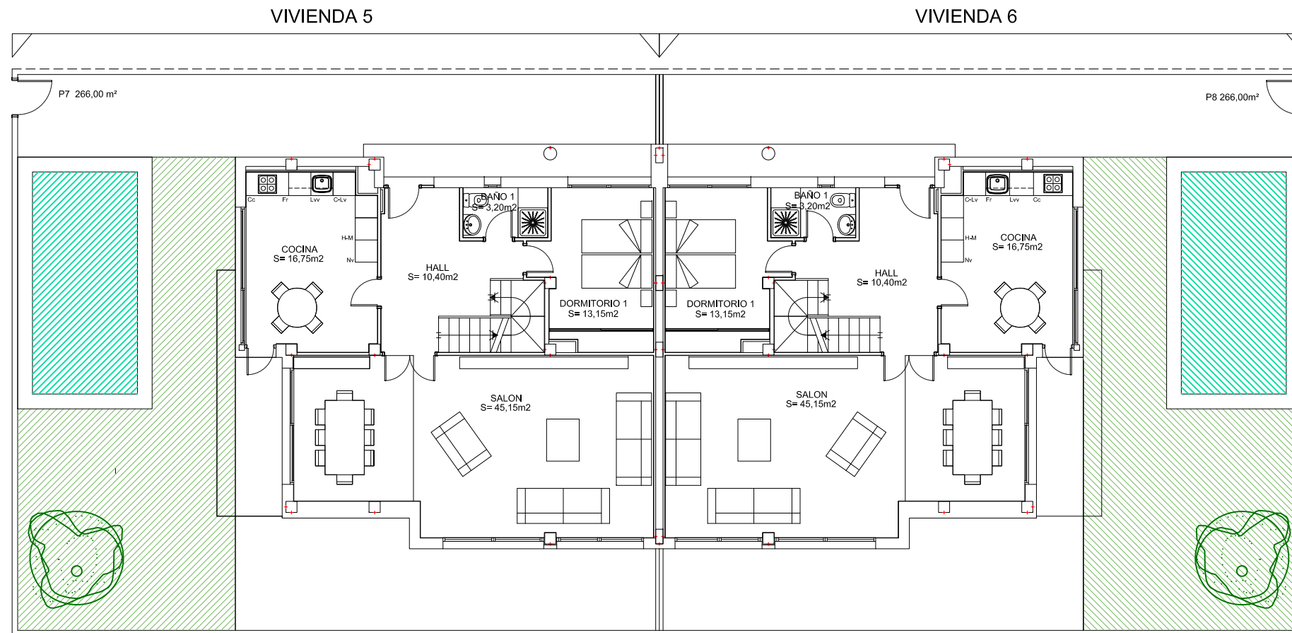
PLANTA BAJA VIVIENDAS 5 Y 6
