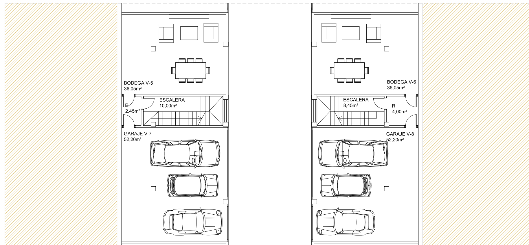
PLANTA SOTANO VIVIENDAS 5 Y 6
