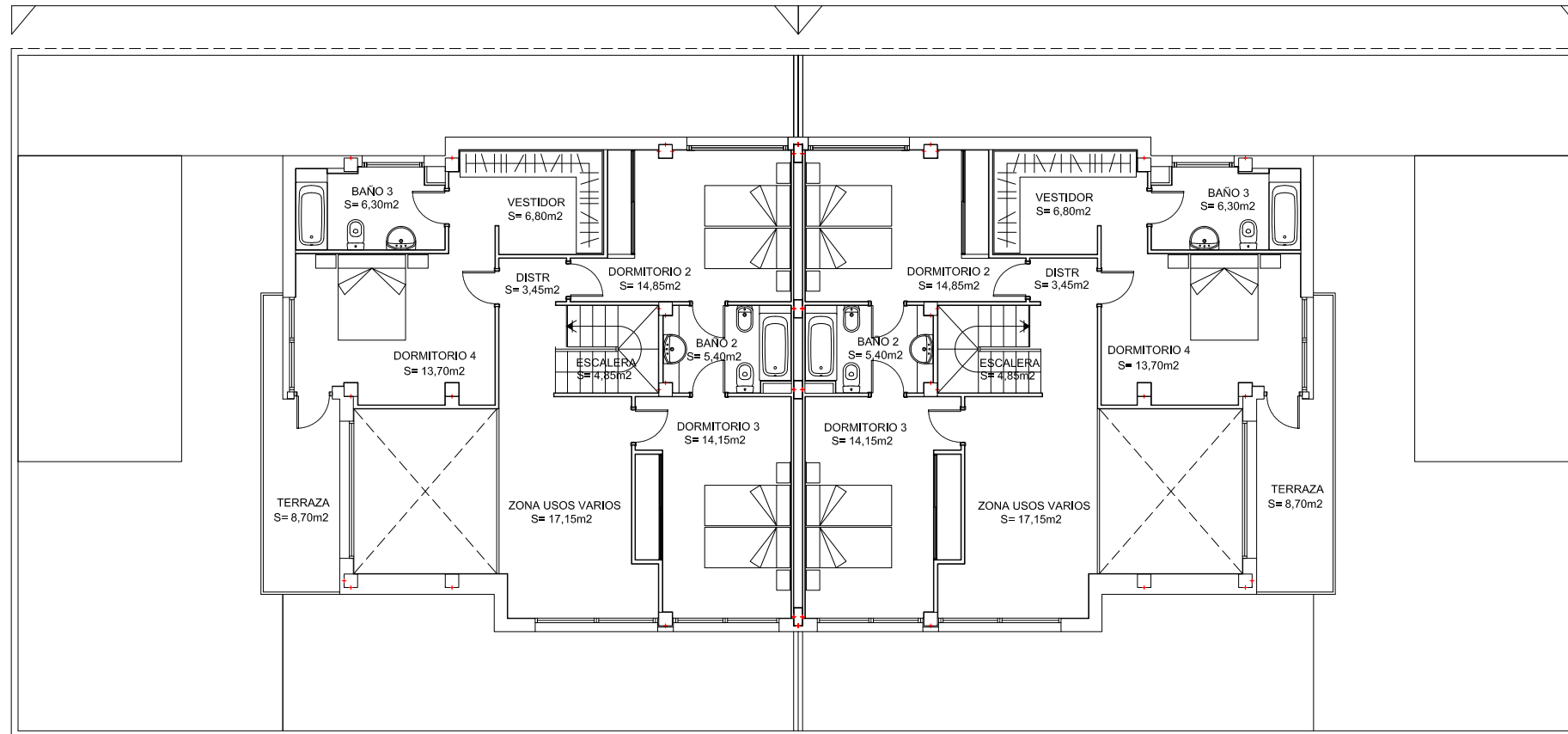
PLANTA PRIMERA VIVIENDAS 5 Y 6
