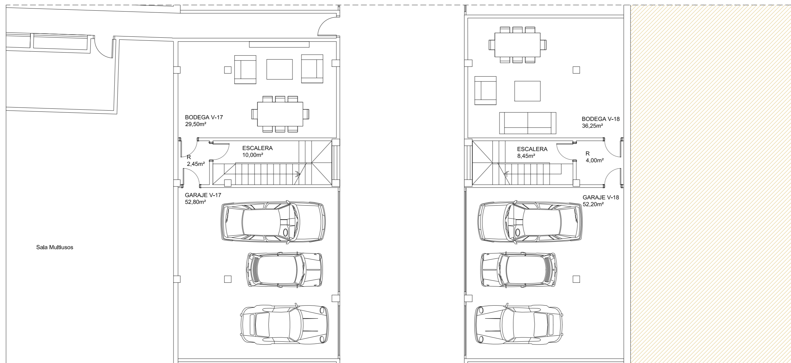
PLANTA SOTANO VIVIENDAS 17 Y 18
