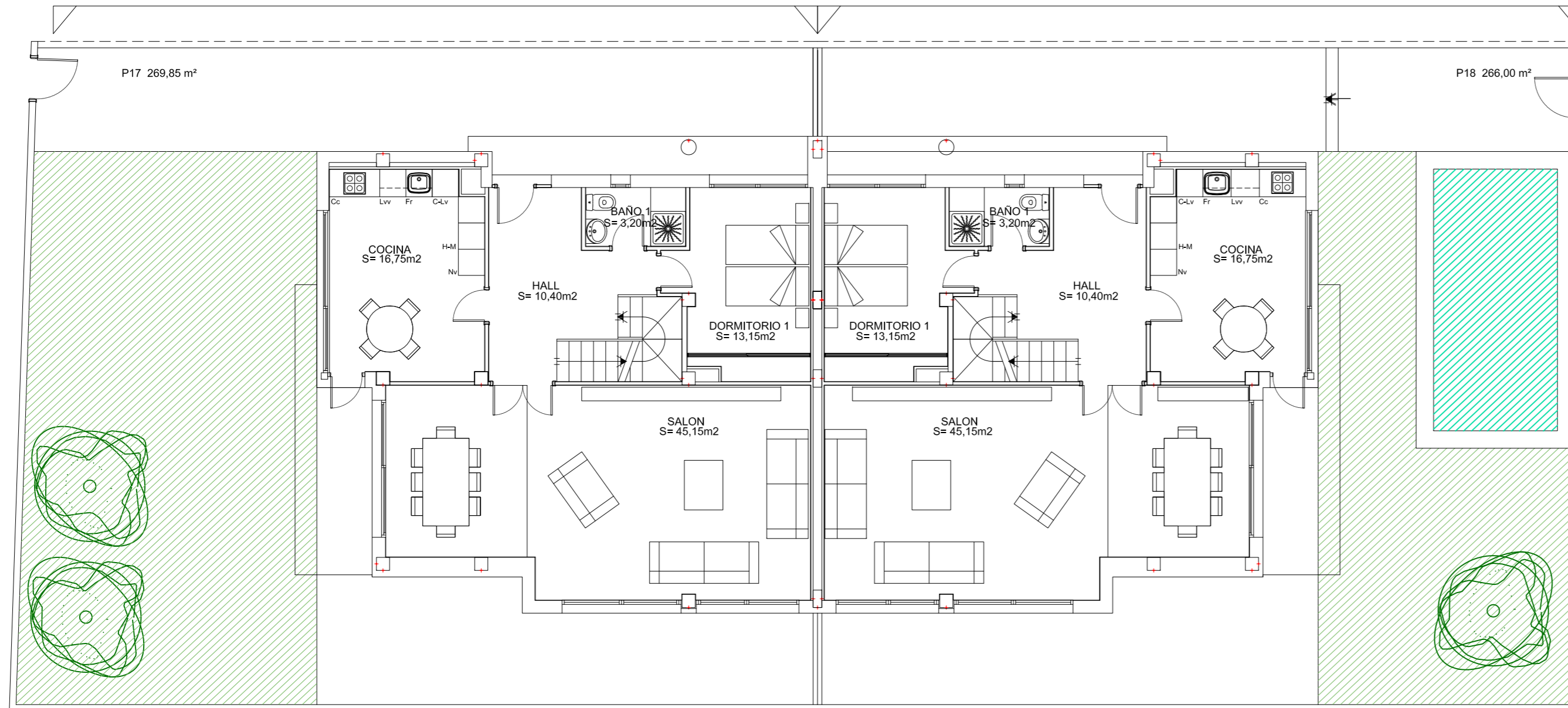
PLANTA BAJA VIVIENDAS 17 Y 18
