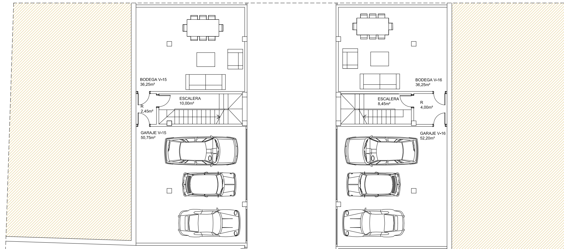
PLANTA SOTANO VIVIENDAS 15 Y 16
