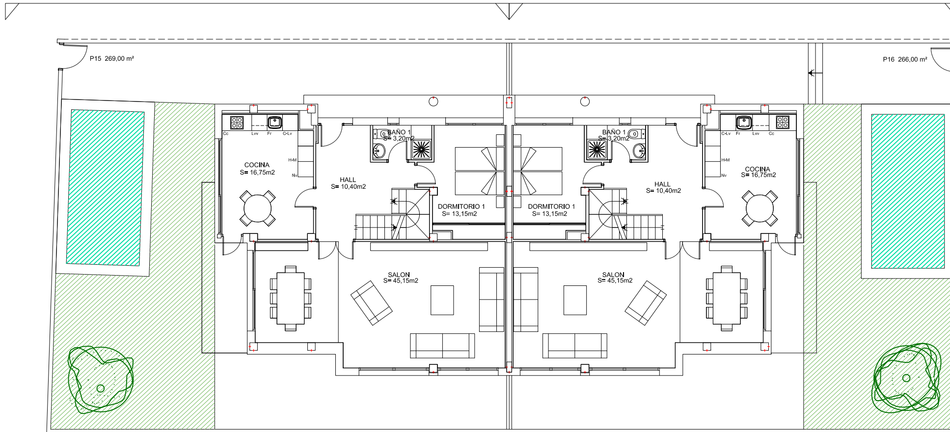
PLANTA BAJA VIVIENDAS 15 Y 16
