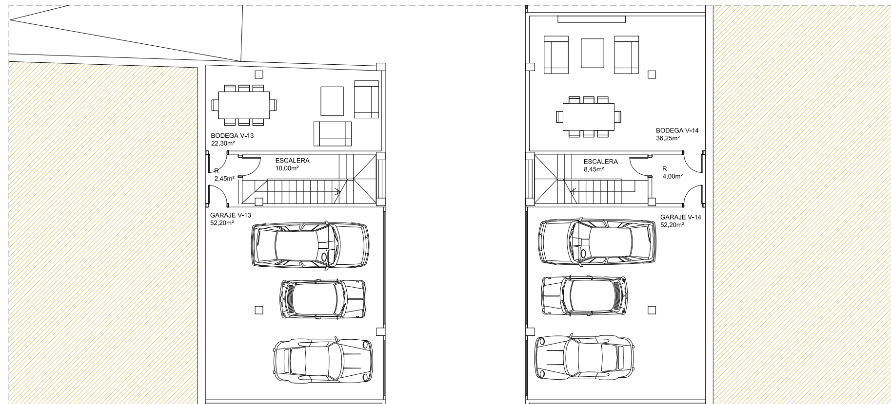
PLANTA SOTANO VIVIENDAS 13 Y 14
