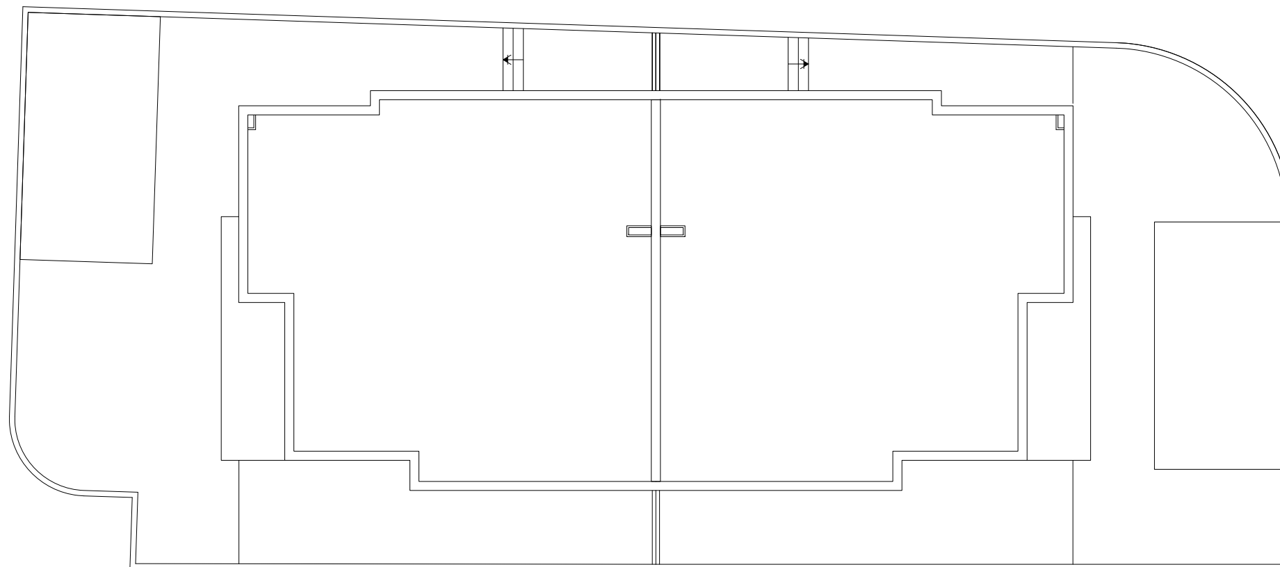
PLANTA CUBIERTAS VIVIENDAS 11 Y 12
