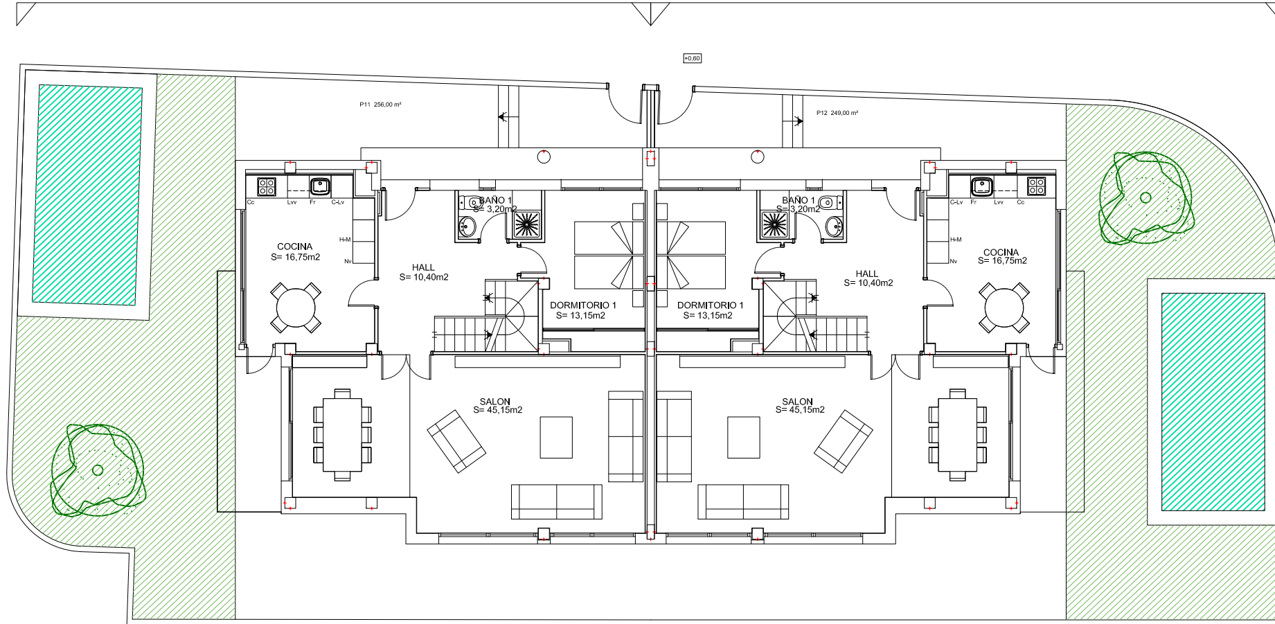
PLANTA BAJA VIVIENDAS 11 Y 12
