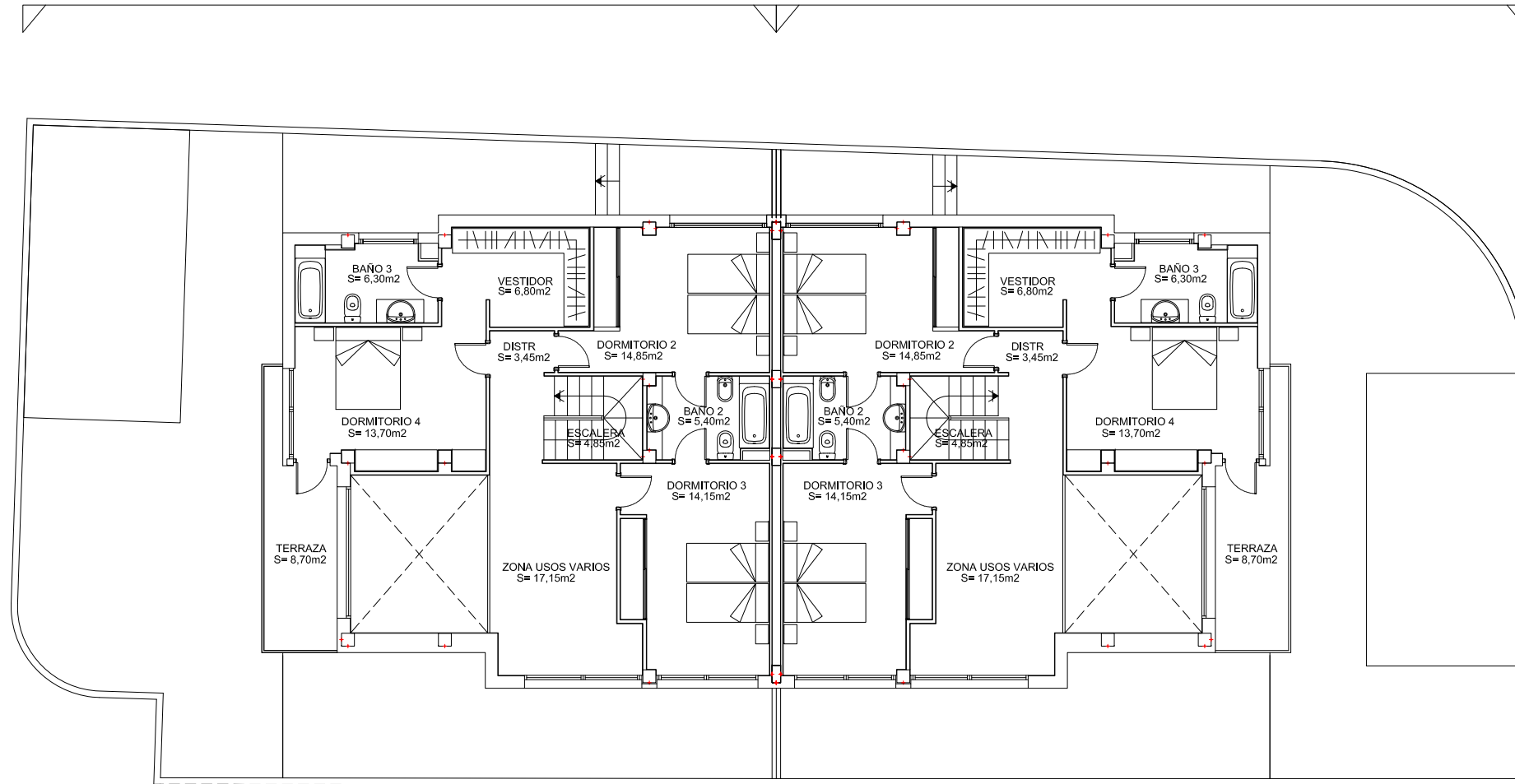
PLANTA PRIMERA VIVIENDAS 11 Y 12
