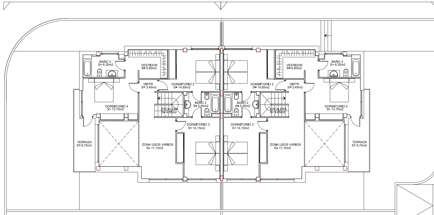
PLANTA PRIMERA VIVIENDAS 1 Y 2
